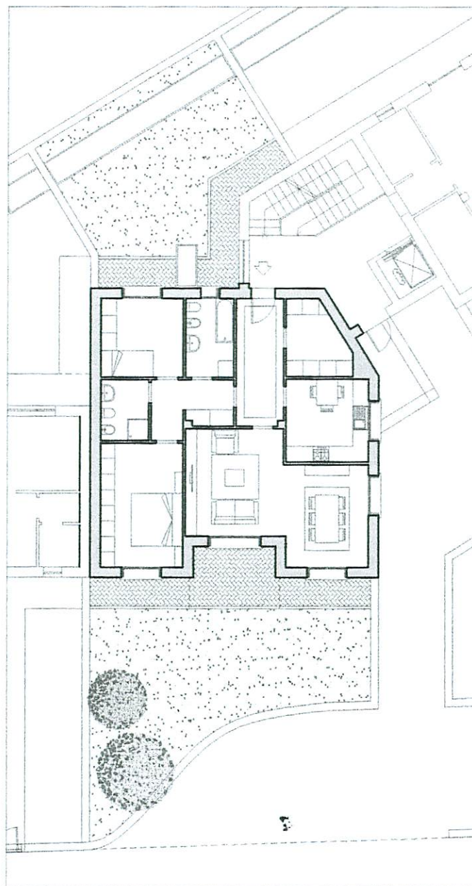
PLANIMETRIA ALLOGGIO E GIARDINO
